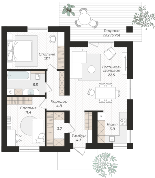
Планировка
