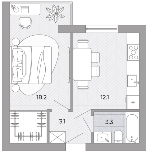
Планировка
